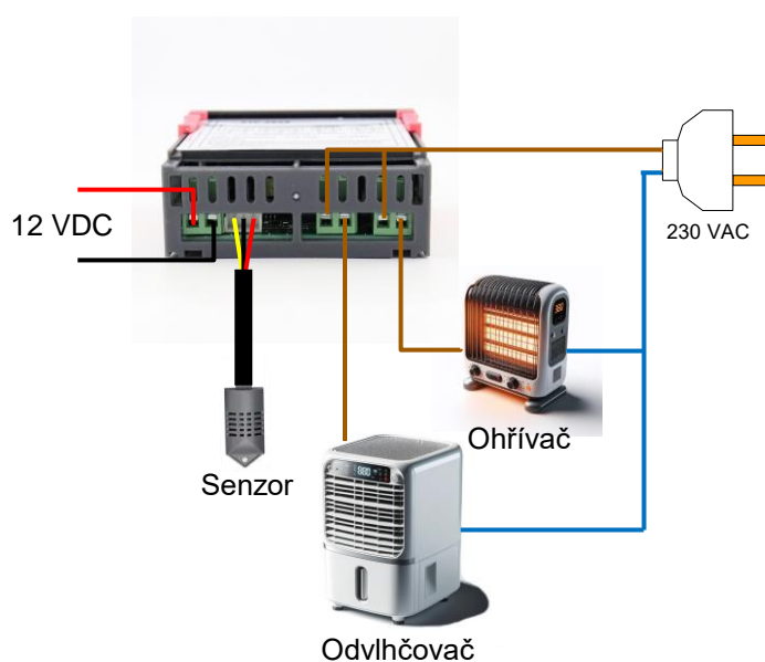
varianta zapojení do sítě
