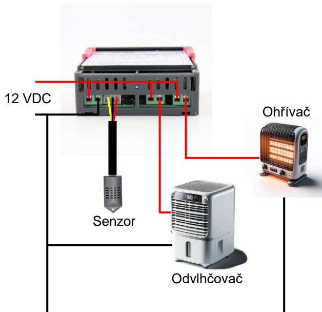
varianta 12V zapojení
